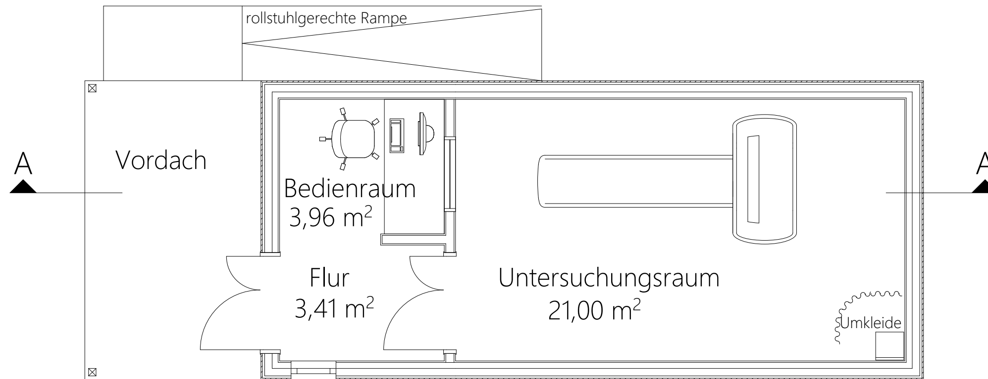
Grundriss
